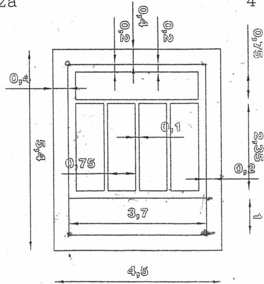
20 posti - 4,50*5,40 5 file in altezza
