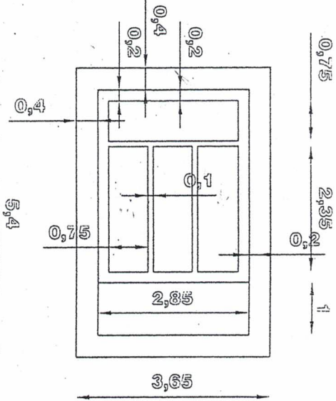
12 posti - 3,65*5,40 4 file in altezza
