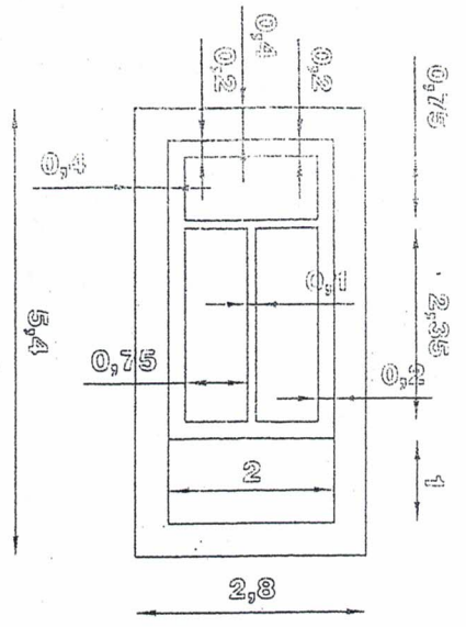
6 posti - 2,80*5,40 3 file in altezza
